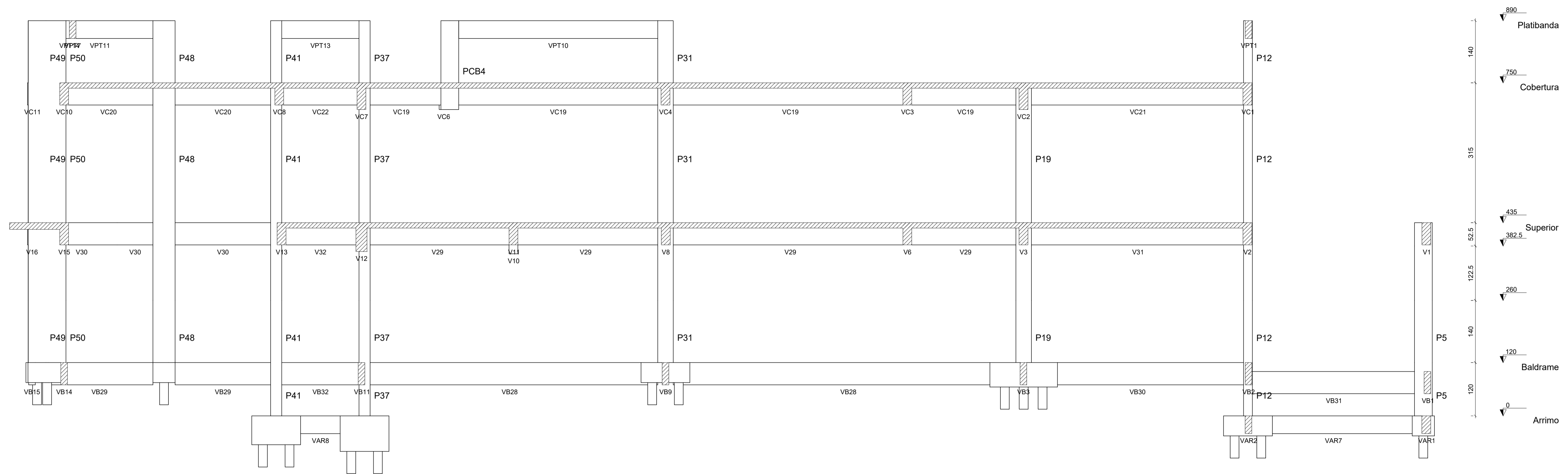
Corte BB Escala 1:50
